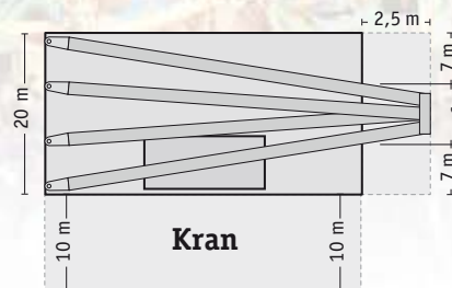
Auf- und Abbauskizze
